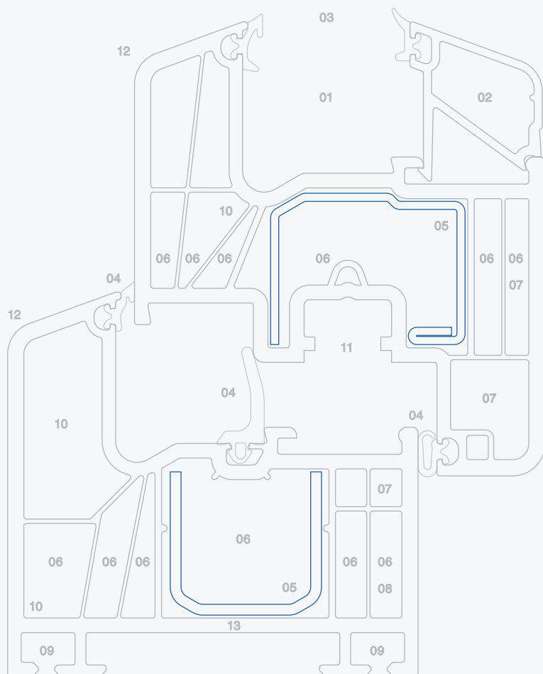
Prestige klasická varianta I 76.6 C2 Těsnění uprostřed (MD)
