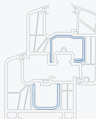
Prestige klasická varianta I 76.6 C2 Těsnění na dorazu (AD)
